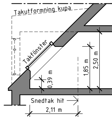
Sektion genom snedtak
